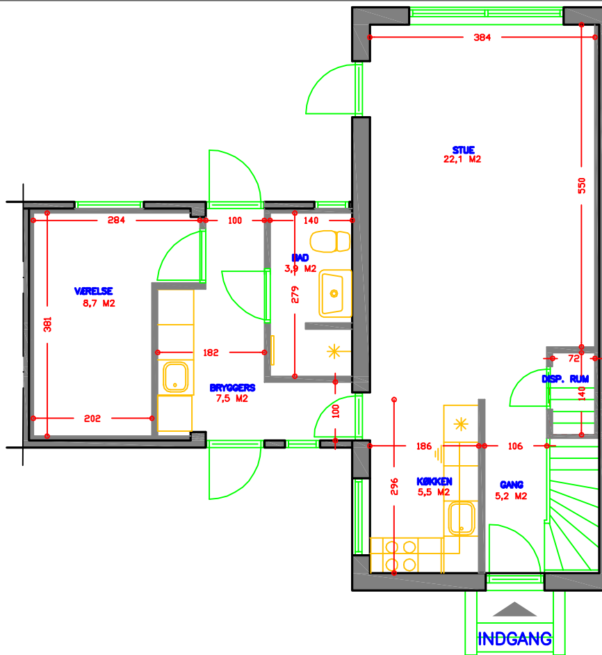
AFDELING 2 TYPE 41 4 RUMS 98 M 2 STUEPLAN
