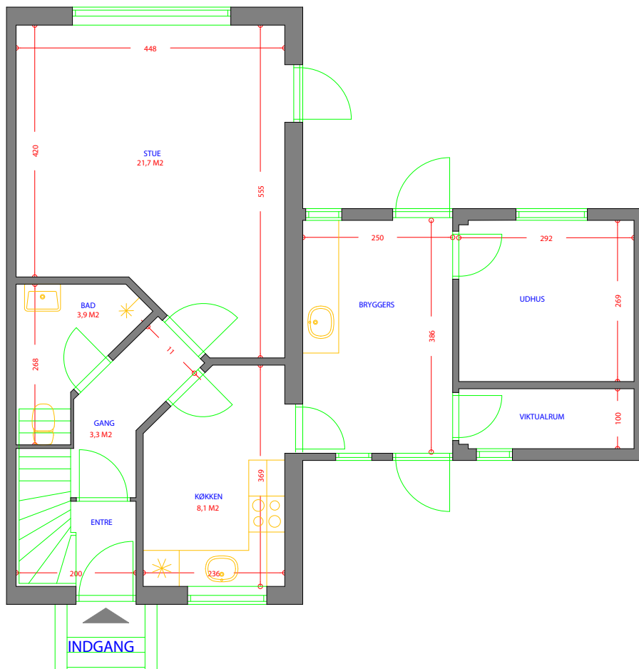
AFDELING 2 TYPE 32 3 RUMS 85 M 2 STUEPLAN
