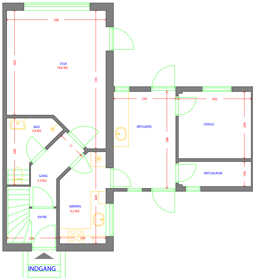
AFDELING 2 TYPE 31 3 RUMS 76 M 2 STUEPLAN
