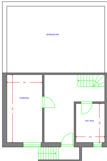
AFDELING 1 TYPE 44 4 RUMS 94M2 KÆLDERPLAN
