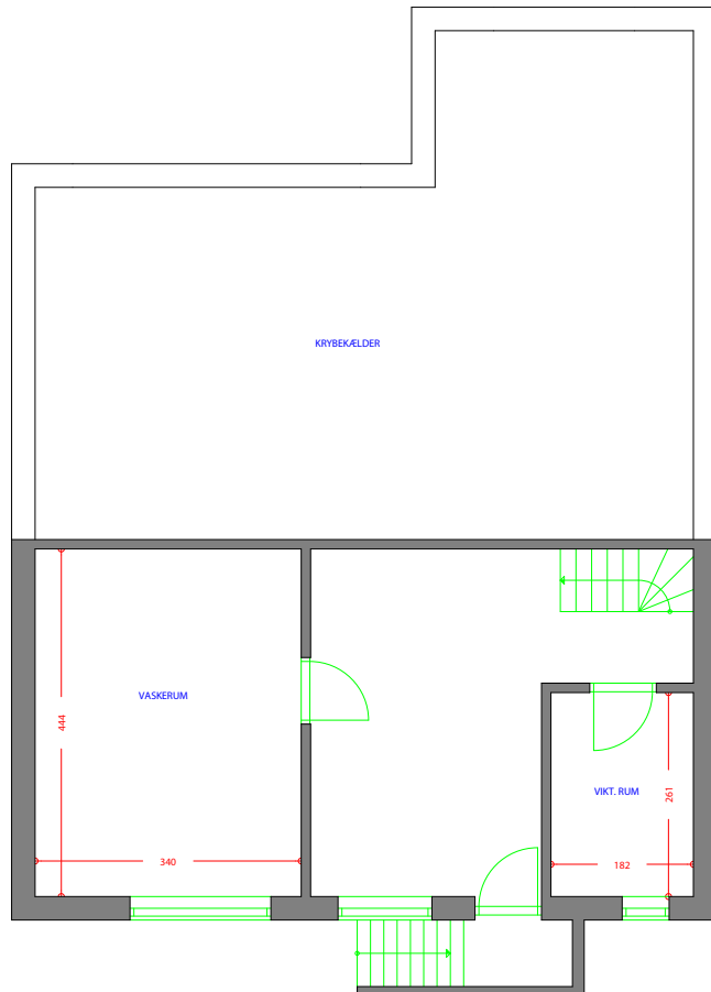
AFDELING 1 TYPE 43 4 RUMS 88M2 KÆLDERPLAN
