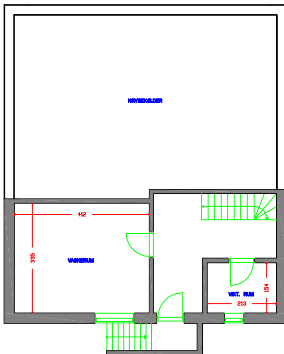
AFDELING 1 TYPE 41 4 RUMS 104M 2 KÆLDERPLAN
