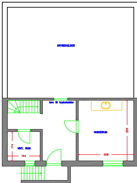
AFDELING 1 TYPE 37 3 RUMS 98 M2 KÆLDERPLAN
