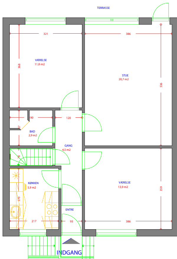
AFDELING 1 TYPE 32 3 RUMS 71M2 STUEPLAN
