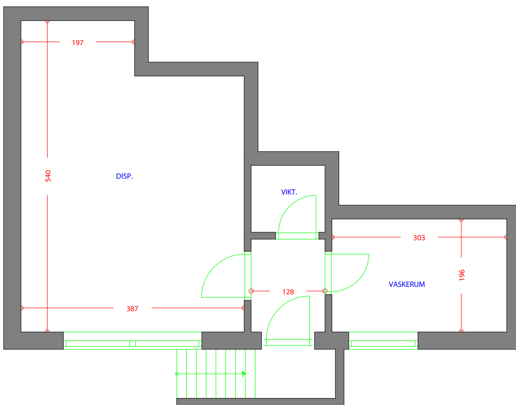
AFDELING 1 TYPE 11 1 RUMS 39M2 KÆLDERPLAN
